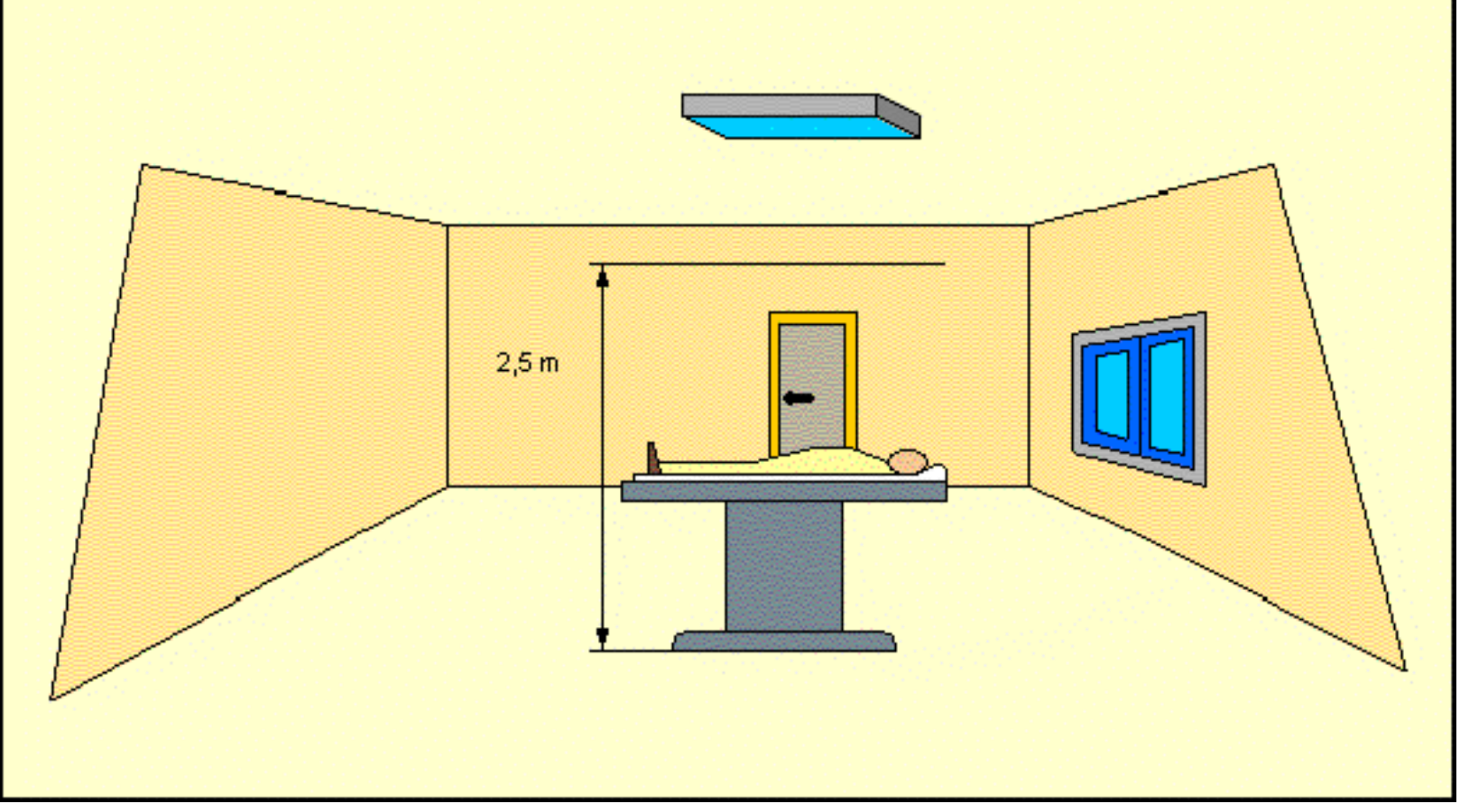
ZONE DI RISPETTO AMBIENTI MEDICI DI TIPO 1
