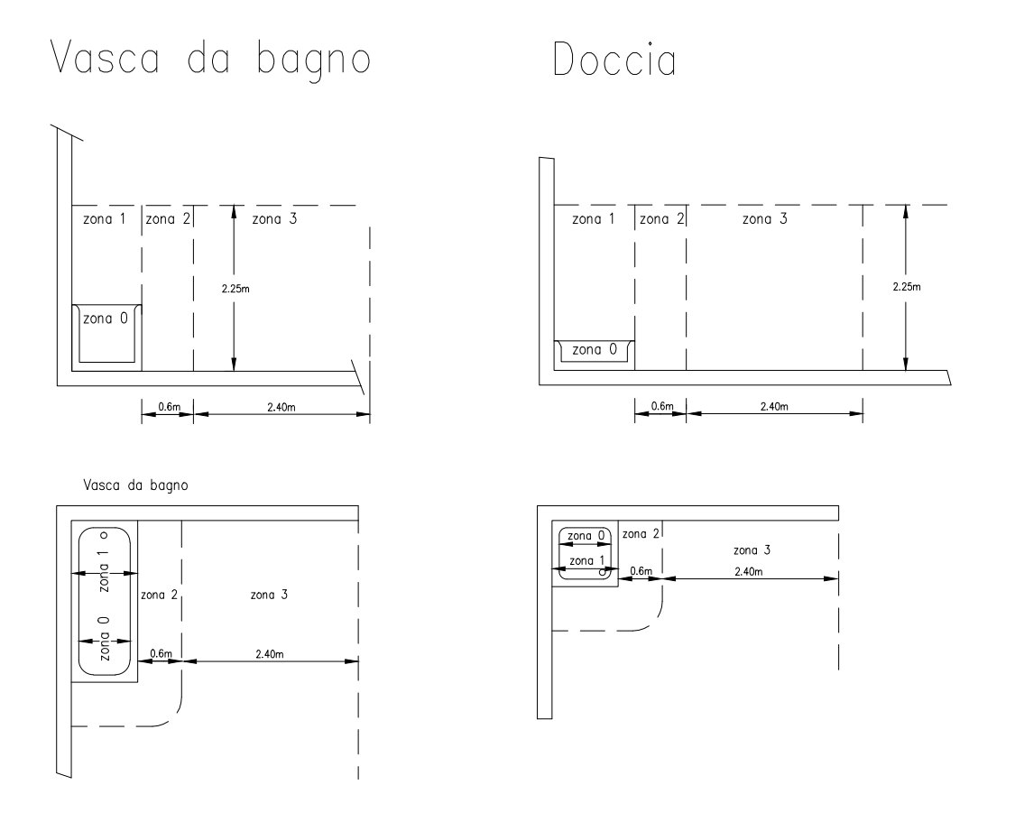
ZONE DI RISPETTO BAGNI PARTICOLARE NON IN SCALA
