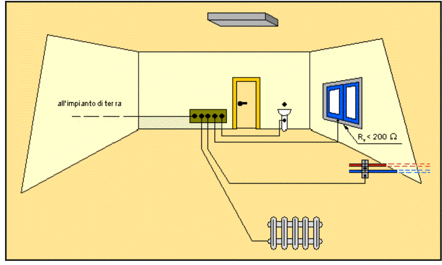
EQUIPOTENZIALITA' AMBIENTI MEDICI DI TIPO 1
