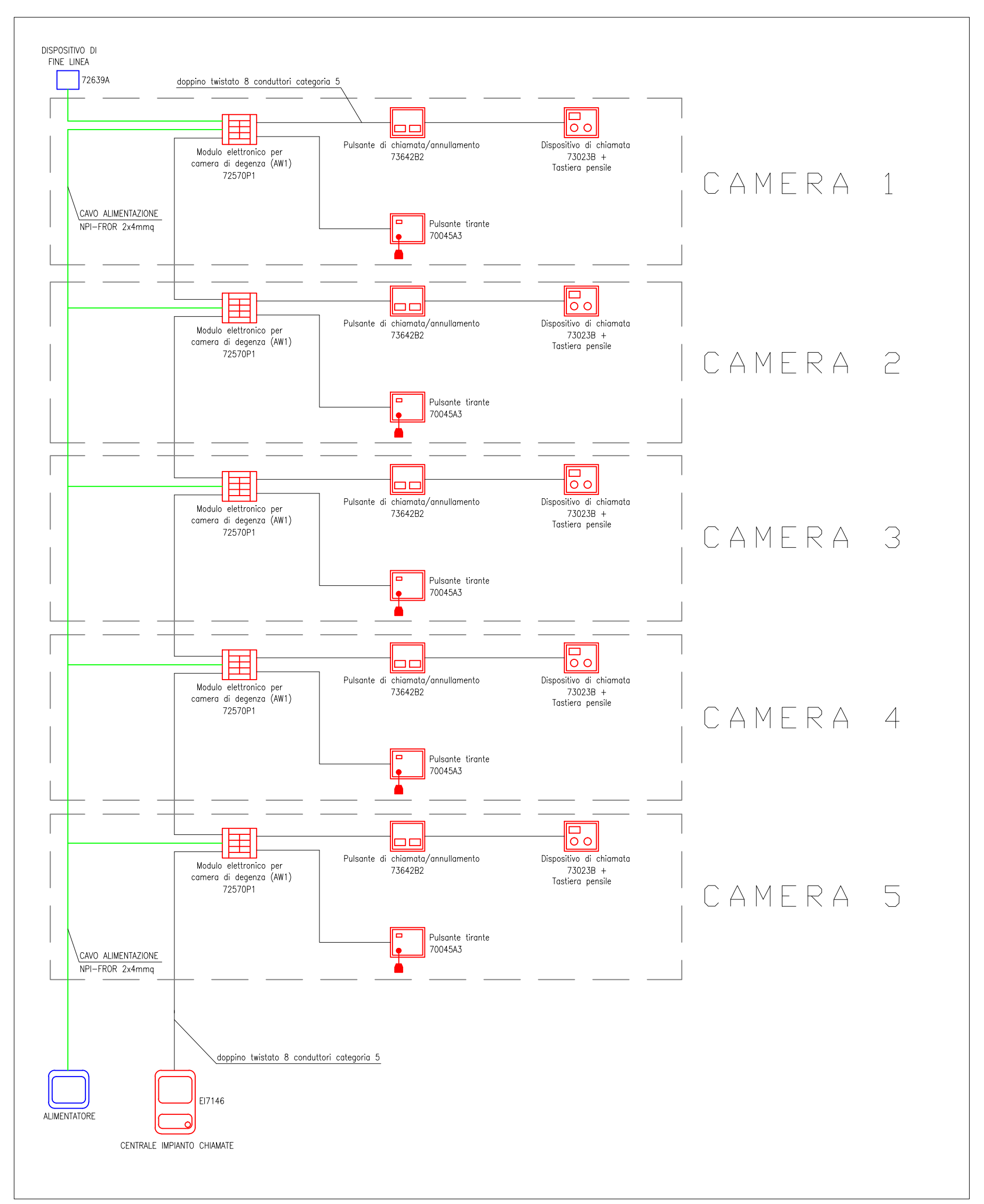
SCHEMA FUNZIONALE IMPIANTO CHIAMATE
